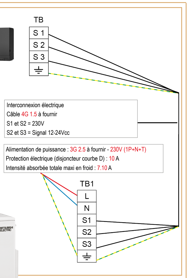
MSZ-EF25VGKB
