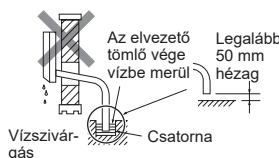
Vízszivárgás Hullámok
