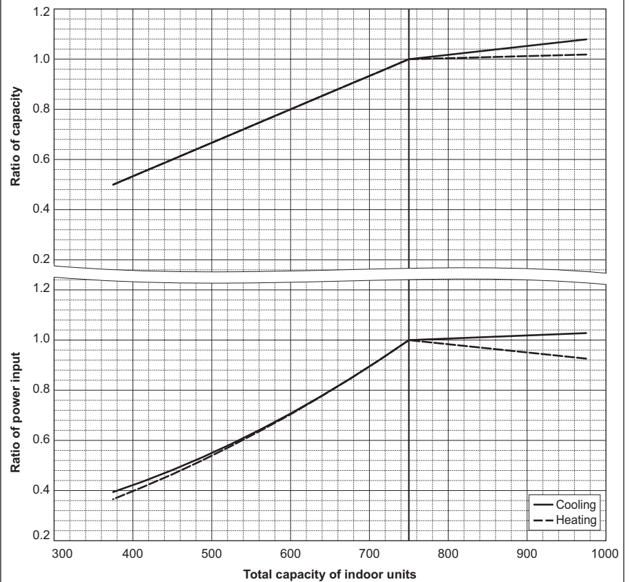
PUHY-EP800YSNW-A2
