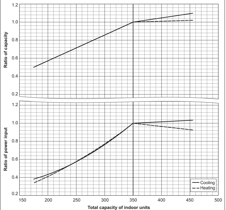
PUHY-EP350YNW-A2
