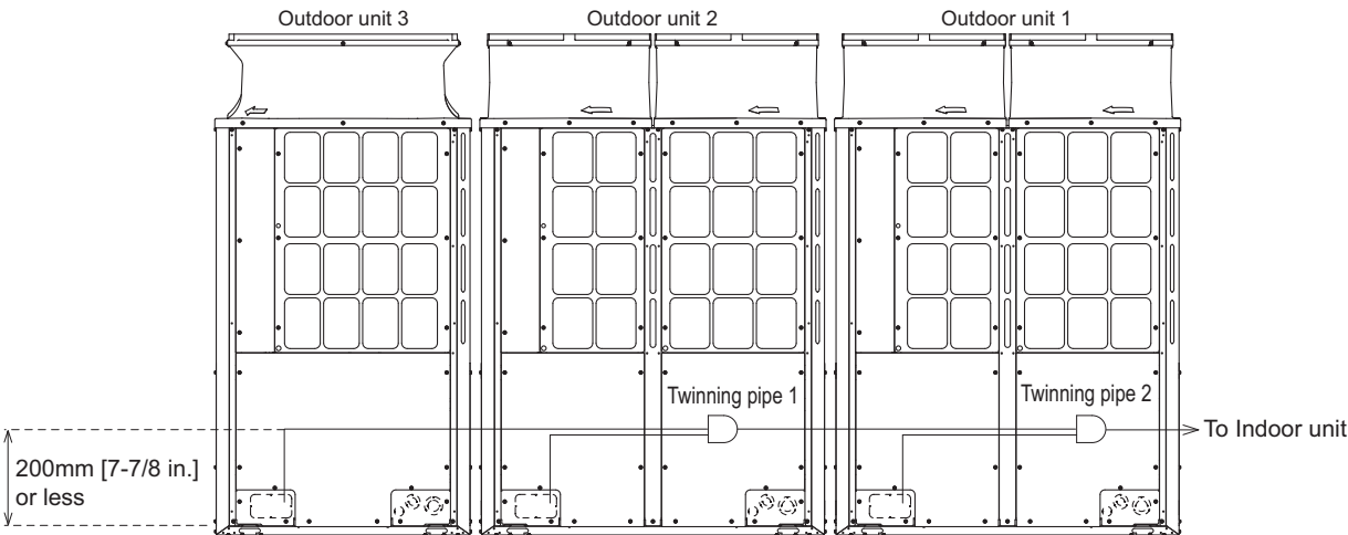
<PUHY-EP950, 1000, 1050YSNW-A2>
