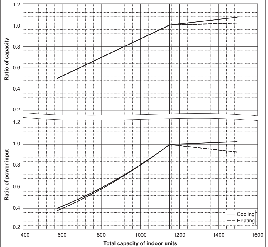
PUHY-EP1200YSNW-A2
