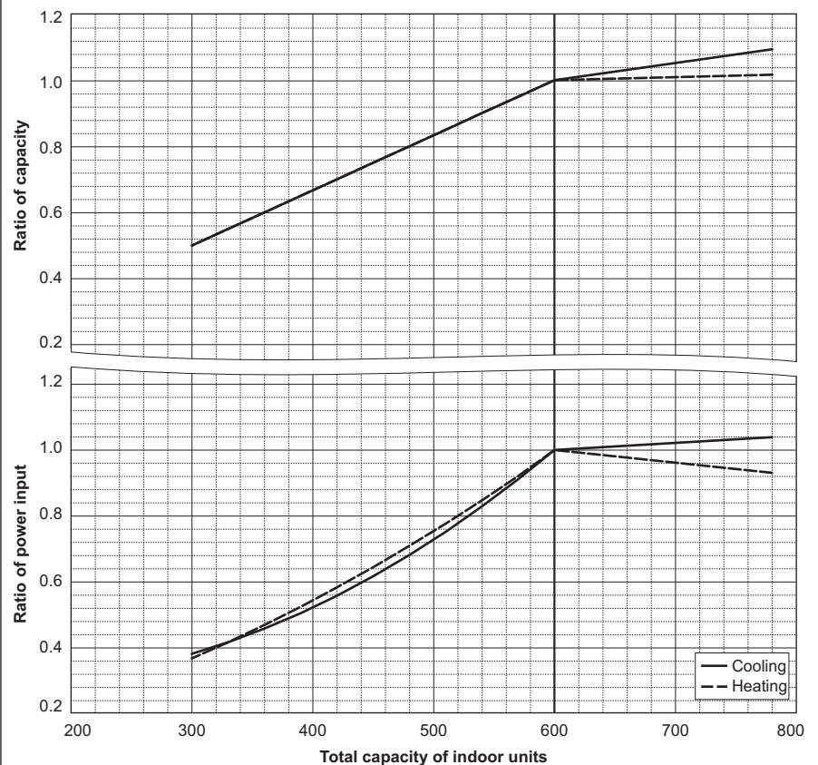
PUHY-EP600YSNW-A2
