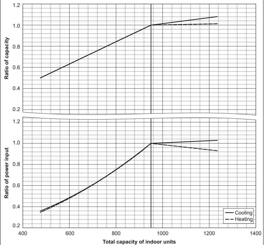
PUHY-EP1000YSNW-A2
