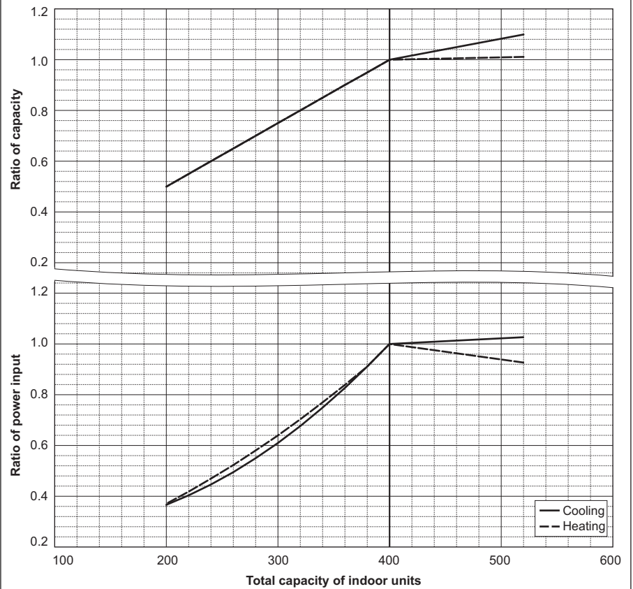
PUHY-EP400YSNW-A2
