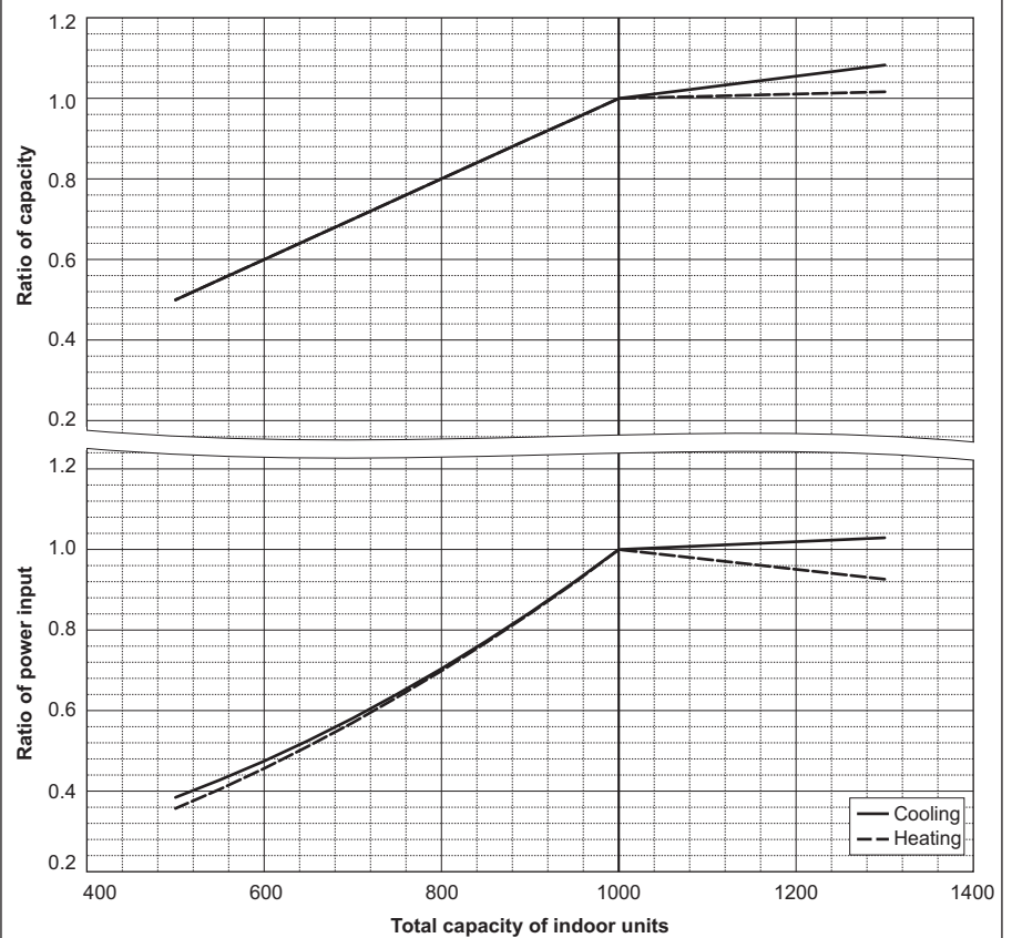
PUHY-EP1000YSNW-A2
