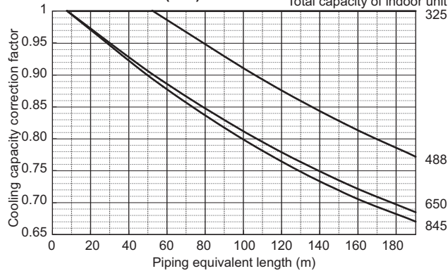
PUHY-EP650YSNW-A2(-BS)
