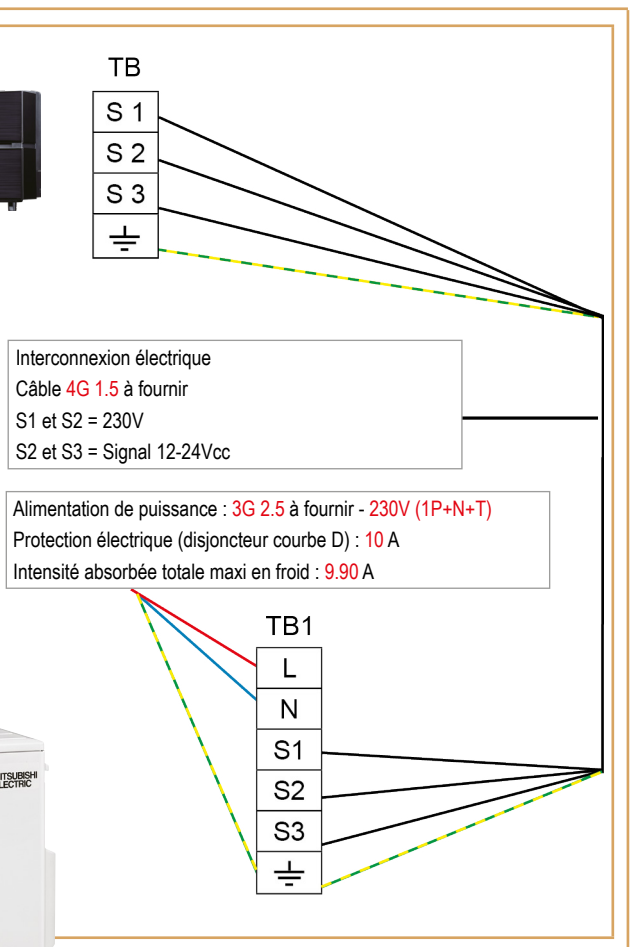
MSZ-LN25VG2B
