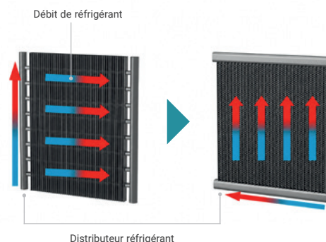
Echangeur classique
