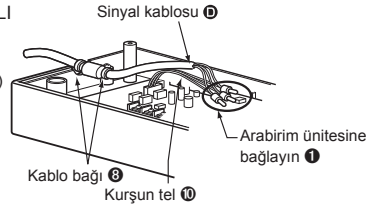
Kart anahtarı bobin zamanlayıcı bağlantısı
