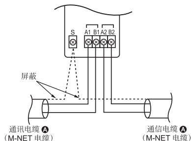
当通信电缆 ① 不是交叉布线时
