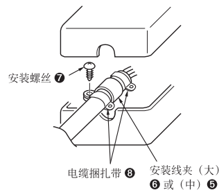
当通信电缆 ① 不是交叉布线时
