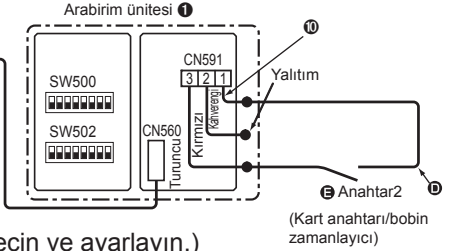
Kart anahtarı bobin zamanlayıcı bağlantısı
