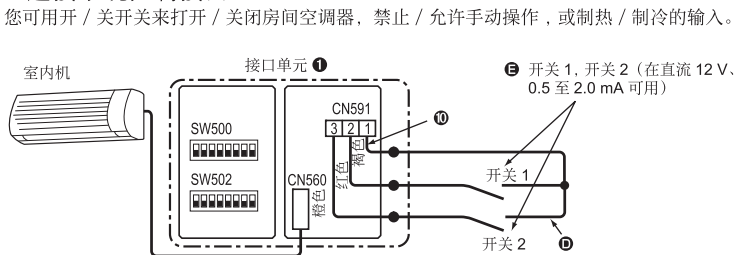
卡片钥匙、纽扣定时器连接
