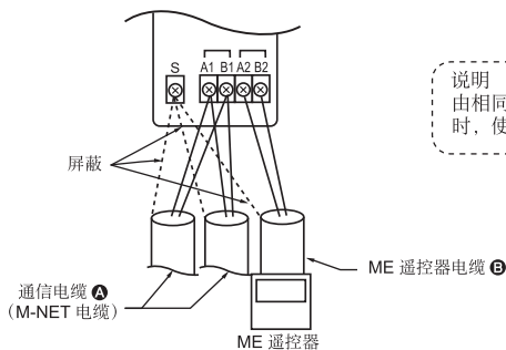
当通信电缆 ① 是交叉布线时
