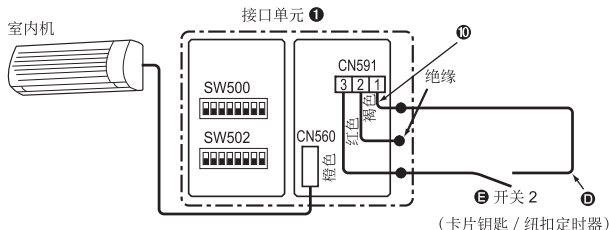
卡片钥匙、纽扣定时器连接
