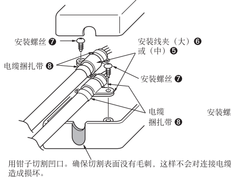
当通信电缆 ① 是交叉布线时
